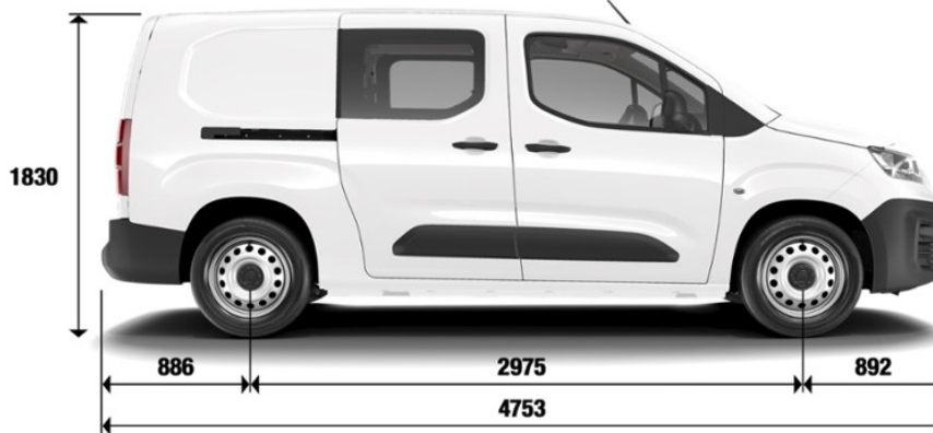
Габаритні розміри, мм
